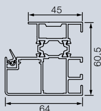
Zárubeň A2
