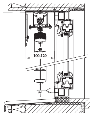
Montáž EXT-50 H do okenního otvoru, provedení s krycím plechem
