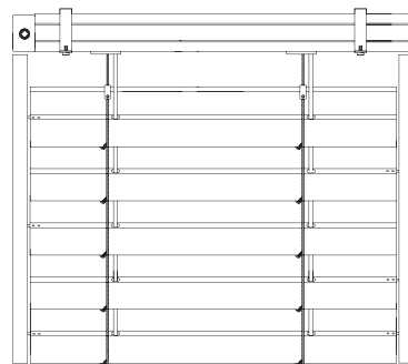
Obr. 1 - boční vedení v lištách
