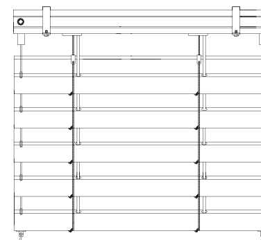
Obr. 2 - boční vedení v lanku
